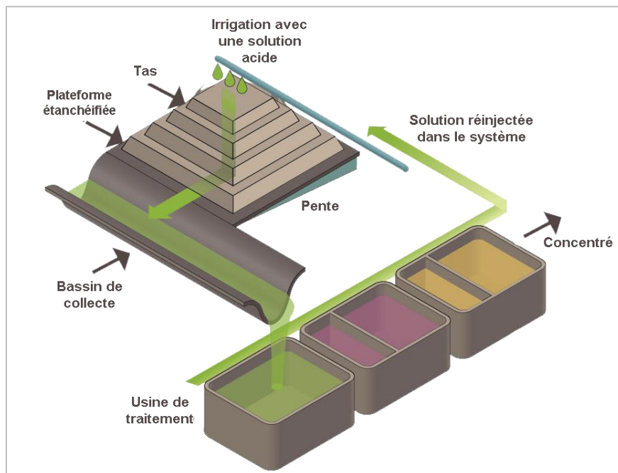
Figure 32 : Schéma de principe de la lixiviation en tas ; adapté et traduit de Nuclear Regulatory Commission · 2017 · cc by 2.0
