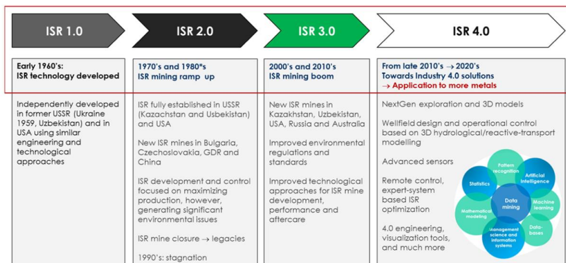
Figure 39 : Aperçu des tendances du développement de la lixiviation in situ entre 1960 et 2020 et description de la lixiviation 4.0 ; tiré de (BIOMore, 2018)
