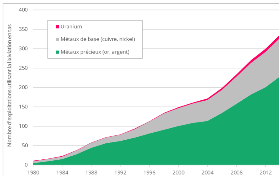
Figure 34 : Démarrage des principales exploitations minières utilisant la lixiviation en tas entre 1980 et 2014 et actuellement en exploitation ; d'après données Intelligence mine dans (Basov, 20/08/2015, Mining.com )
