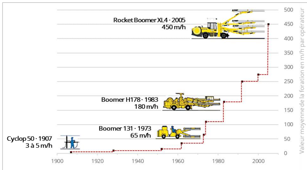
Figure 23 : Développement de la foration par opérateur, en mètres par heure, de 1905 à 2005 ; adapté de Atlas Copco Rocks Drills, 2005 ; dans (Zare & Bruland, 2007)
