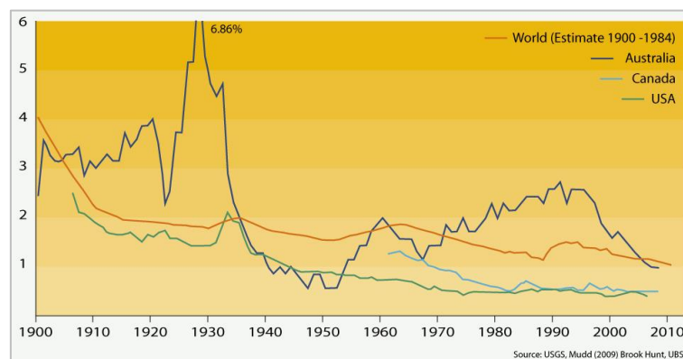
Figure 17 : Évolution globale des teneurs en cuivre, de 1900 à 2010 par GRID-Arendal · cc by-nc-sa 2.0 ; tiré de (GRID-Arendal, 2014)
