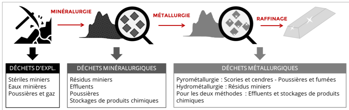
Figure 5 : Représentation schématique des principaux déchets solides, liquides et gazeux associés aux processus d'exploitation et de traitement du minerai | SystExt · Septembre 2021 · cc by-sa-nc 3.0
