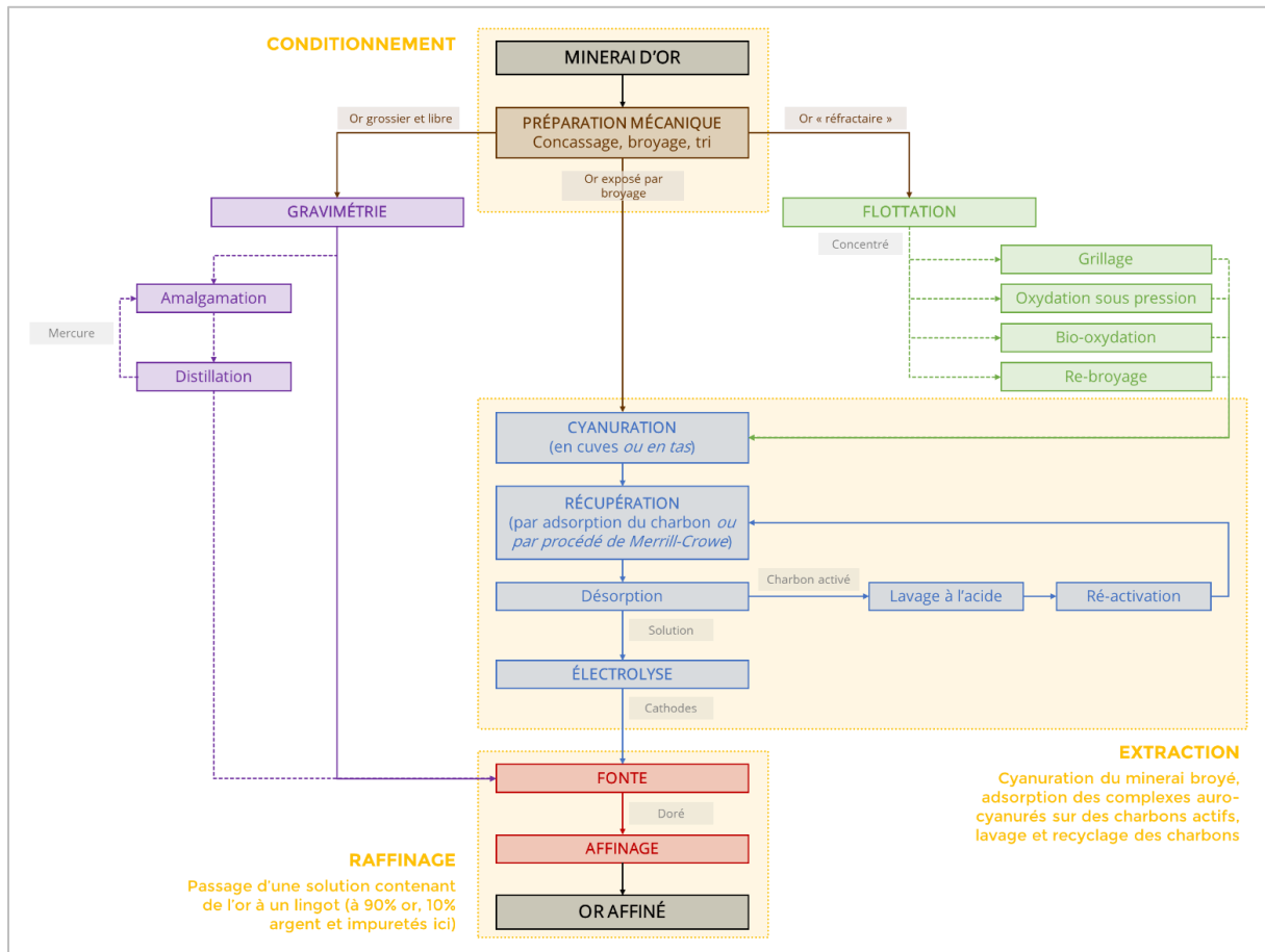
Figure 4 : Étapes de traitement qui peuvent être appliquées à un minerai d'or ; tiré de (SystExt, 2020a)
