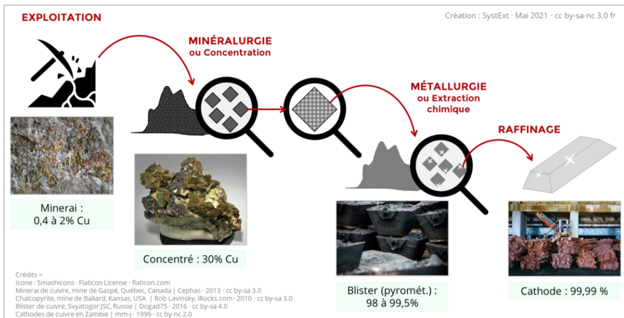
Figure 3 : Représentation schématique des principales étapes de traitement d'un minerai métallique et illustration avec l'exemple du cuivre | SystExt · Mai 2021 · cc by-sa-nc 3.0
