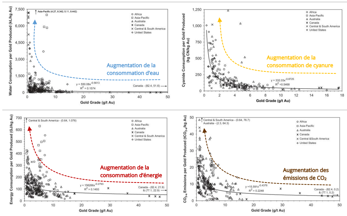
Figure 19 : Évolution de la consommation d'eau, de cyanure, d'énergie et des émissions de CO 2 en fonction de la teneur en or ; tiré de (Mudd, 2007a)
