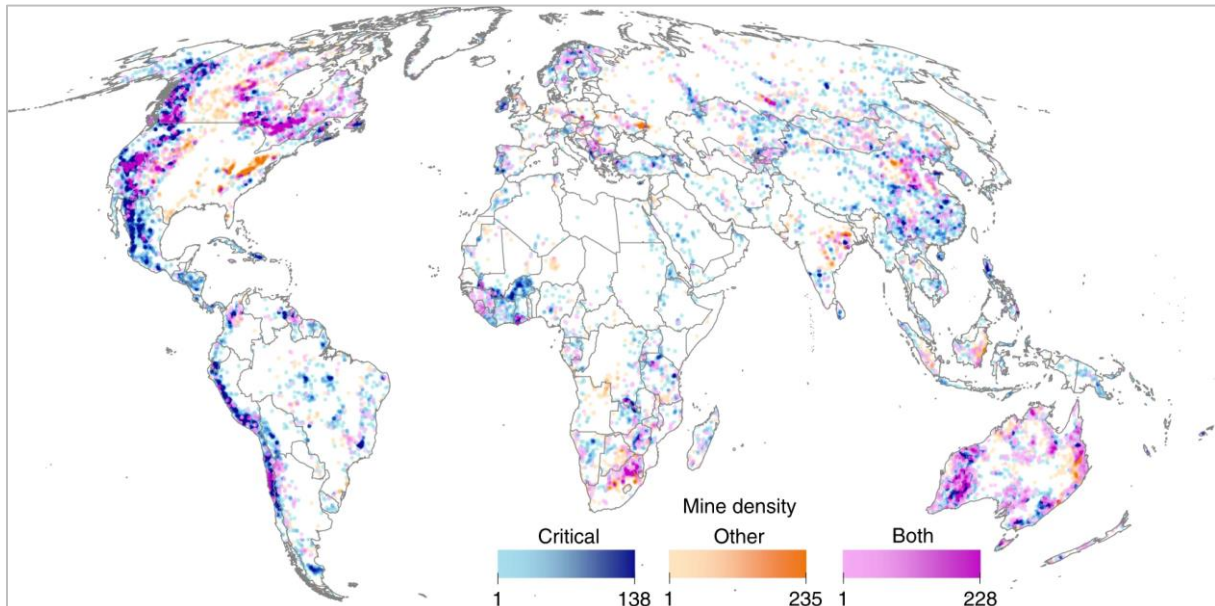
Figure 22 : Carte mondiale des zones minières (mines en phase pré-opérationnelle, en activité et fermées) qui exploitent des métaux nécessaires aux technologies et aux infrastructures des énergies renouvelables ( critical , en bleu), d'autres métaux ( other , en orange) et ces deux types de métaux ( both , en rose), et mise en évidence de la densité associée (en nombre de sites, couleur plus ou moins foncée) ; tiré de (Sonter, et al., 2020, p. 2)
