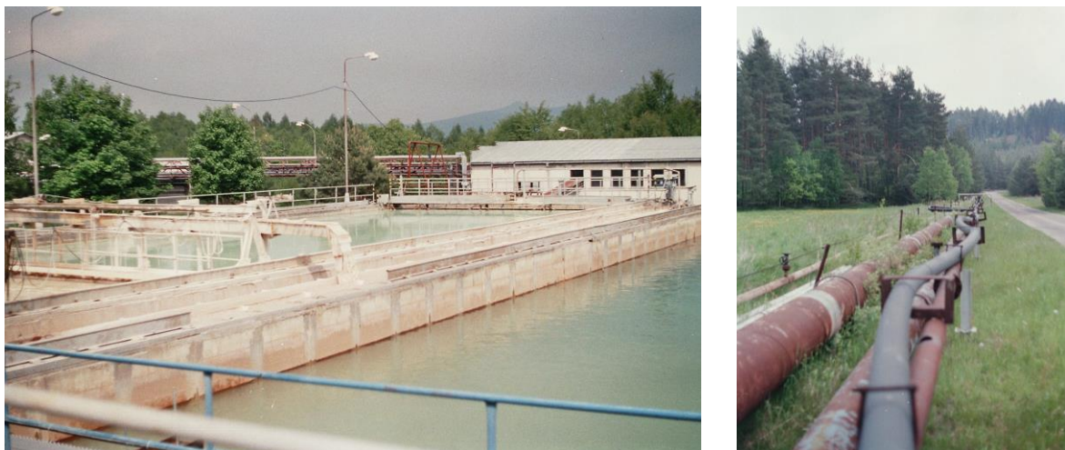
Figure 38 : Ancienne mine d'uranium de Stráž pod Ralskem, République Tchèque, exploitée par lixiviation in situ et par travaux miniers souterrains ; à gauche : usine de traitement et bassins, à droite : conduites de transport des solutions et lixiviats | Jan Helebrant · 2006 · domaine public
