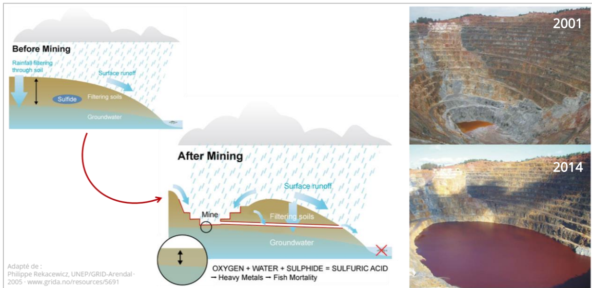
Figure 6 : (à gauche) Eaux minières et mécanismes de pollution en métaux et métalloïdes ; adapté de Philippe Rekacewicz · cc by-sa-nc 2.0 ; tiré de (GRID-Arendal, 2005b) ; (à droite) Mine à ciel ouvert d'Atalaya, (mine de cuivre-or-argent de Rio-Tinto, Espagne) pendant l'exhaure (2001) et après l'arrêt de celui-ci (2014) ; tiré de (Olias & Nieto, 2015, p. 306)
