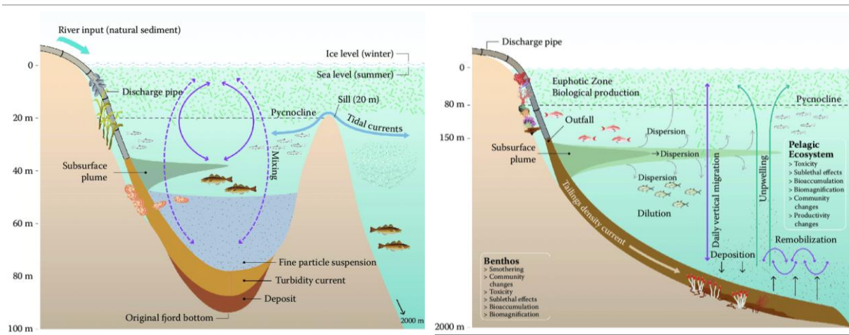
Figure 43 : Représentation des impacts environnementaux associés aux déversements en milieu marin, avec en fjord (à gauche) et en milieu marin profond (à droite) ; tiré de (Morello, et al., 2016, pp. 320-321)
