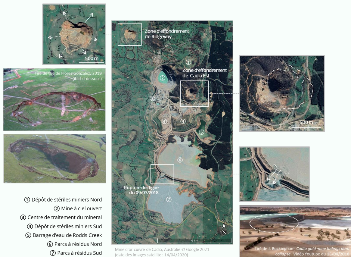
Figure 26 : Situation de la mine d'or cuivre de Cadia, Australie, zones d'effondrement et rupture de digue du 09/03/2018 | Création : SystExt · Octobre 2021
