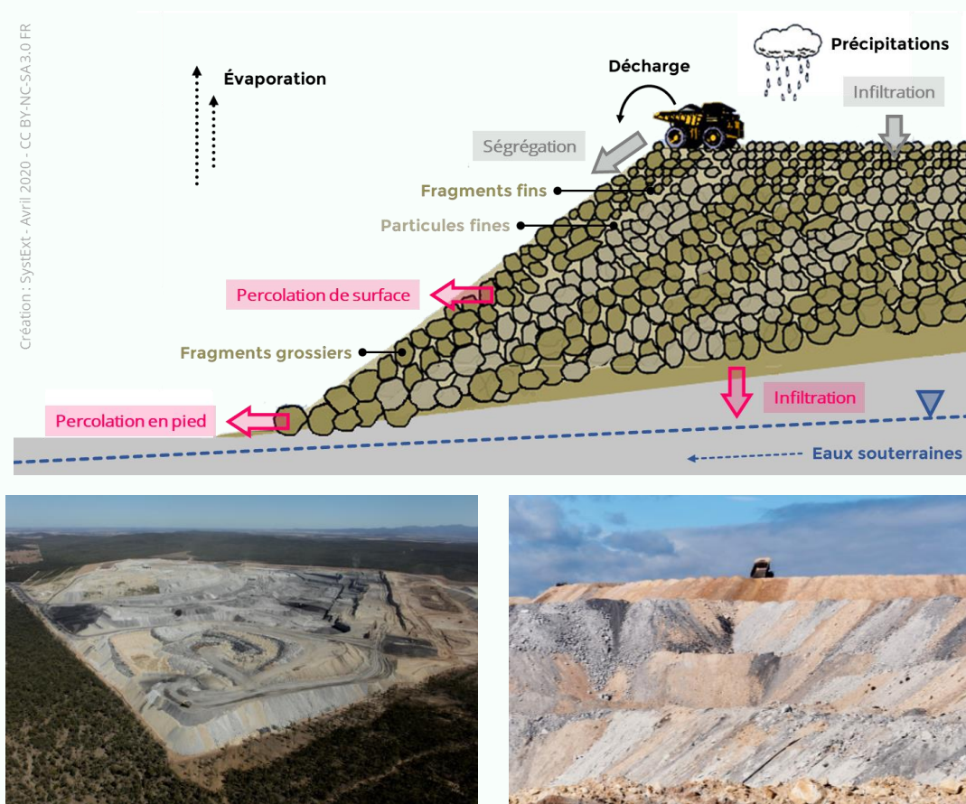
Figure 7 : Principales caractéristiques des dépôts de stériles miniers
