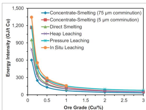
Figure 18 : Consommation énergétique de la production de cuivre en fonction de la teneur du minerai et de la technique de traitement* ; tiré de (Northey, et al., 2014, p. 191)
